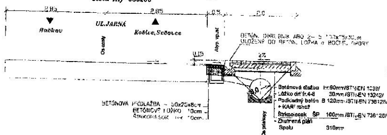
VZOROVÝ PRIEČNY REZ CHODNÍKOM Cesta III/ 050208 M:1:50
